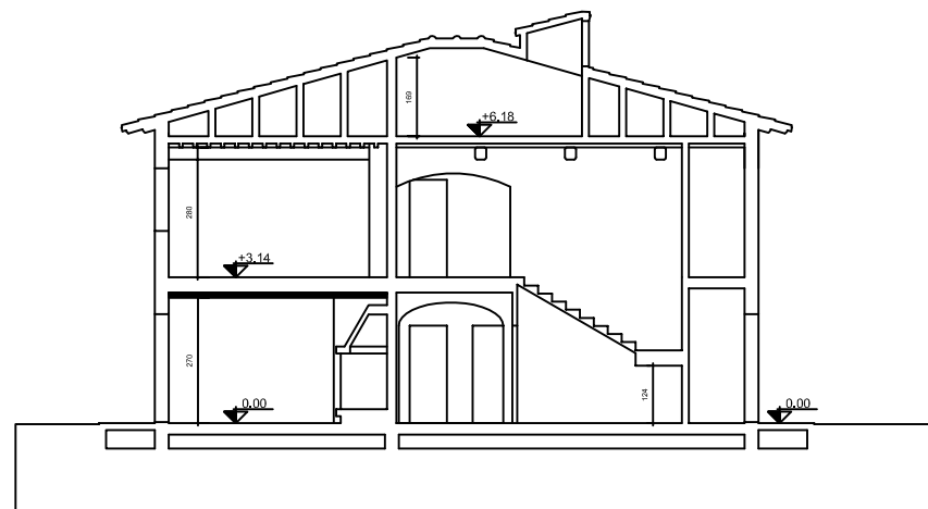
SEZIONE A - B
