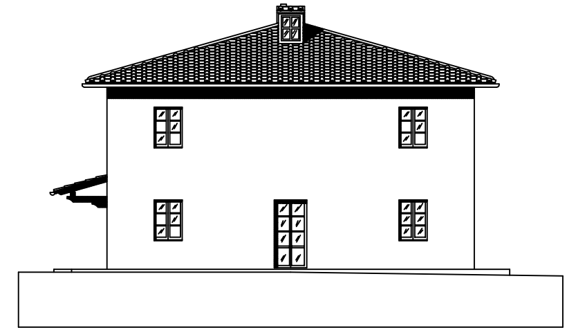
PROSPETTO SUD - EST
