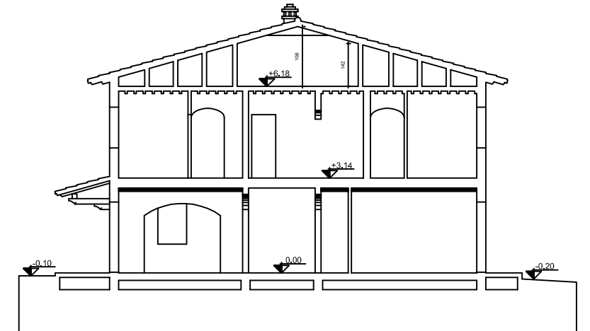
SEZIONE C - D
