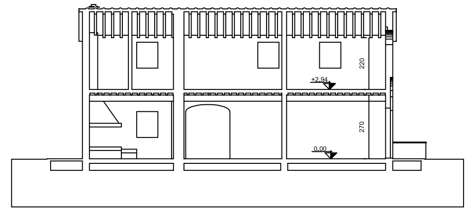
SEZIONE A - B
