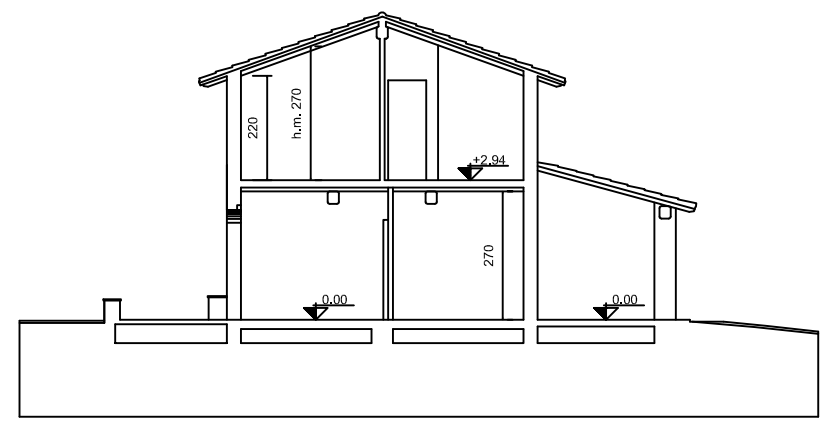
SEZIONE C - D
